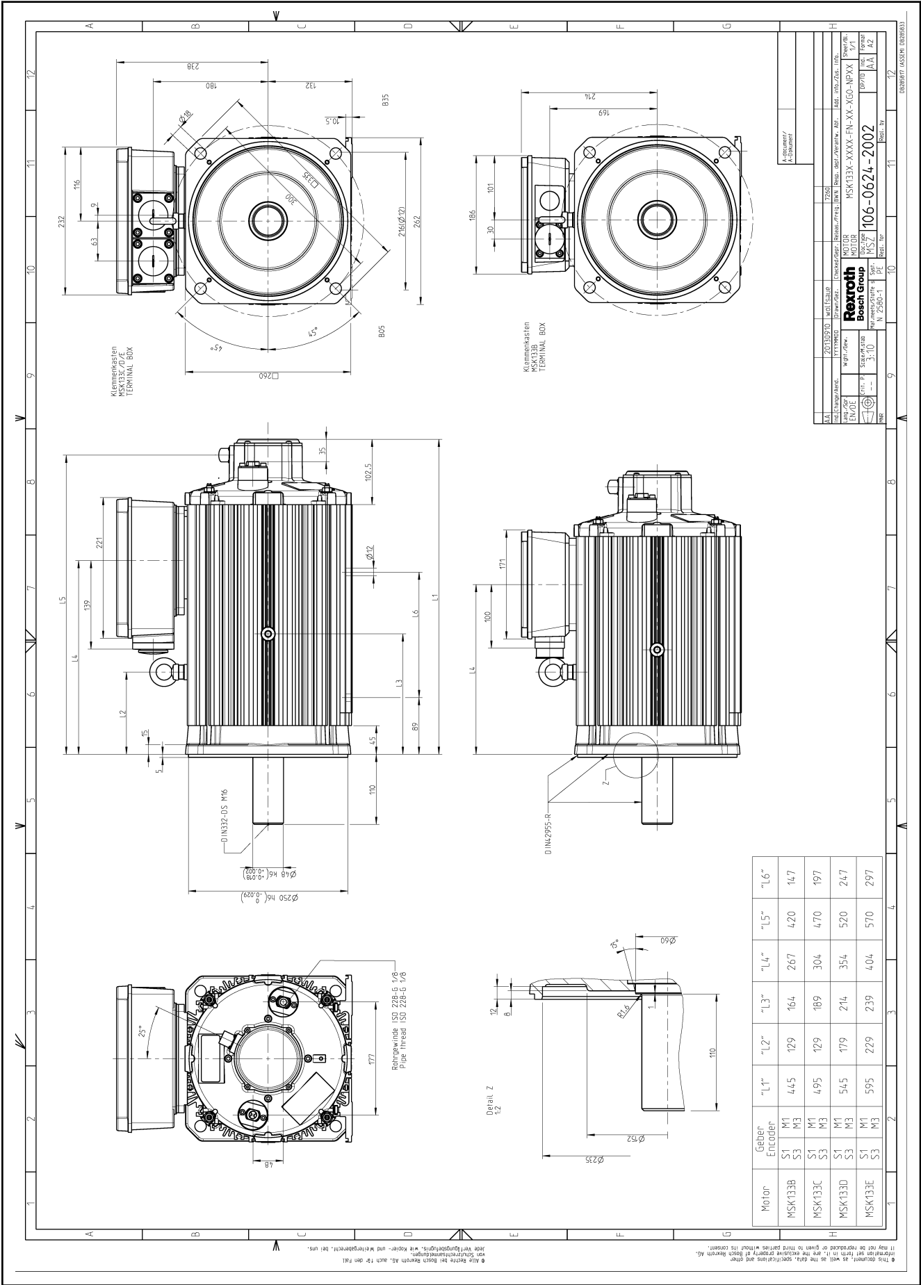
Fig. 5-36: MSK133 - -FN
