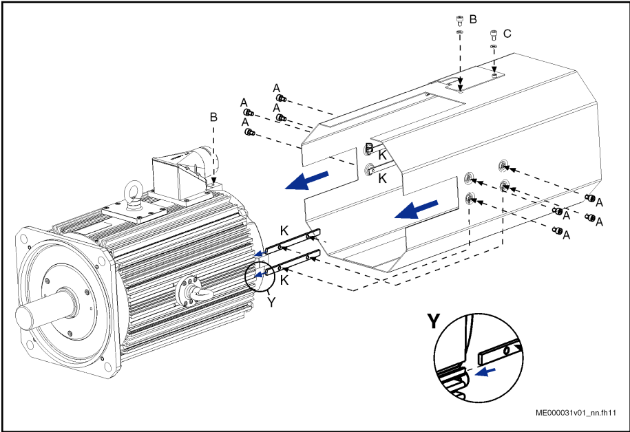
Fig. 7-8: Assembly Fan Unit Axial, Flange Dimension 260
