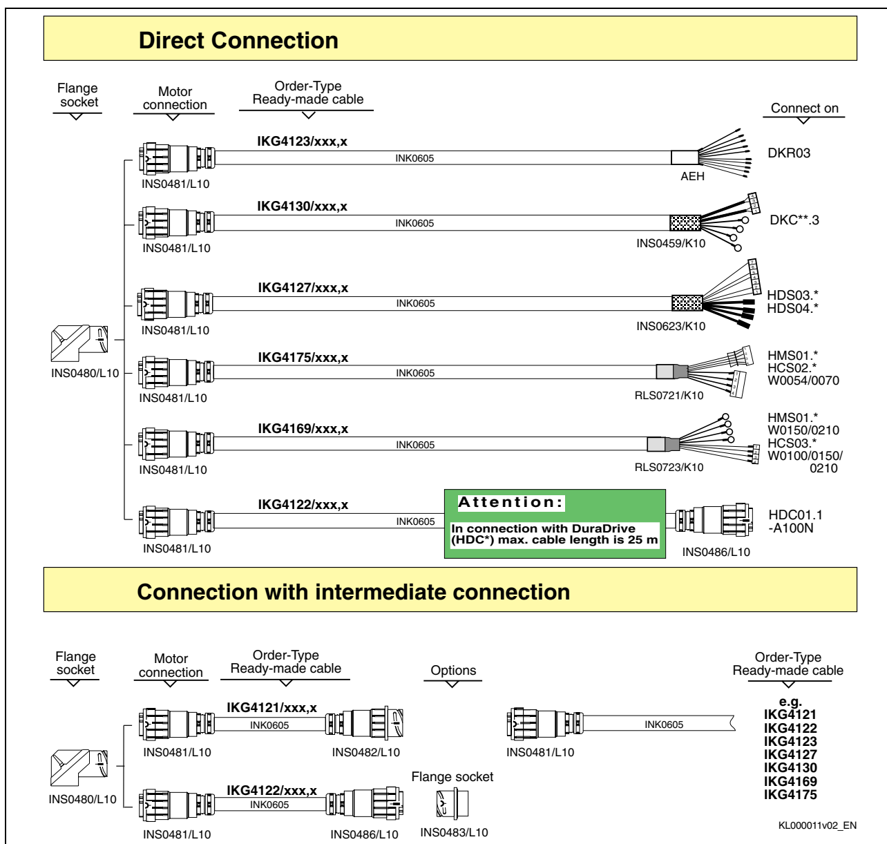
Fig. 17-8: Kabelauswahl INS0480 – 10,0mm 2
