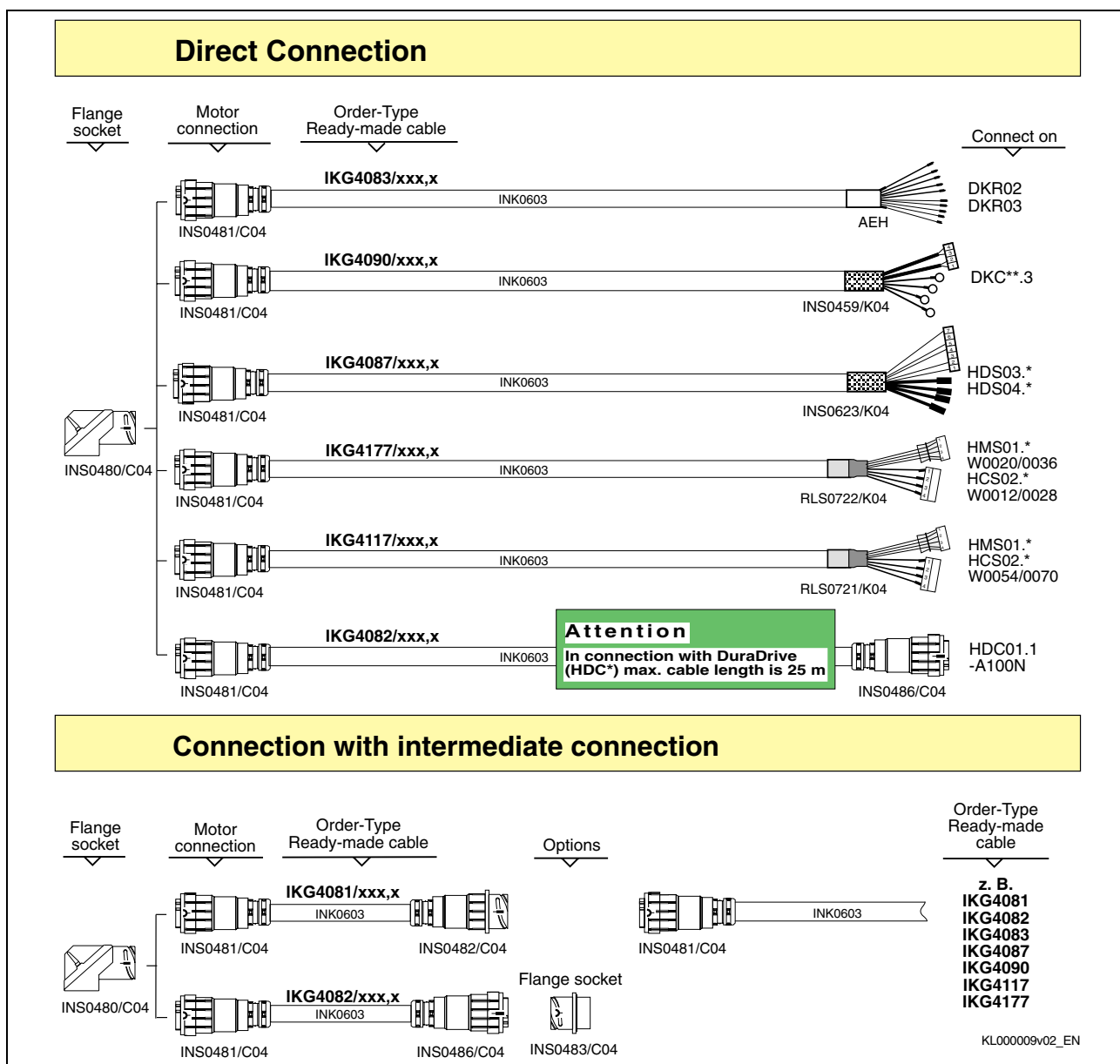
Fig. 17-6: Kabelauswahl INS0480 – 4,0mm 2
