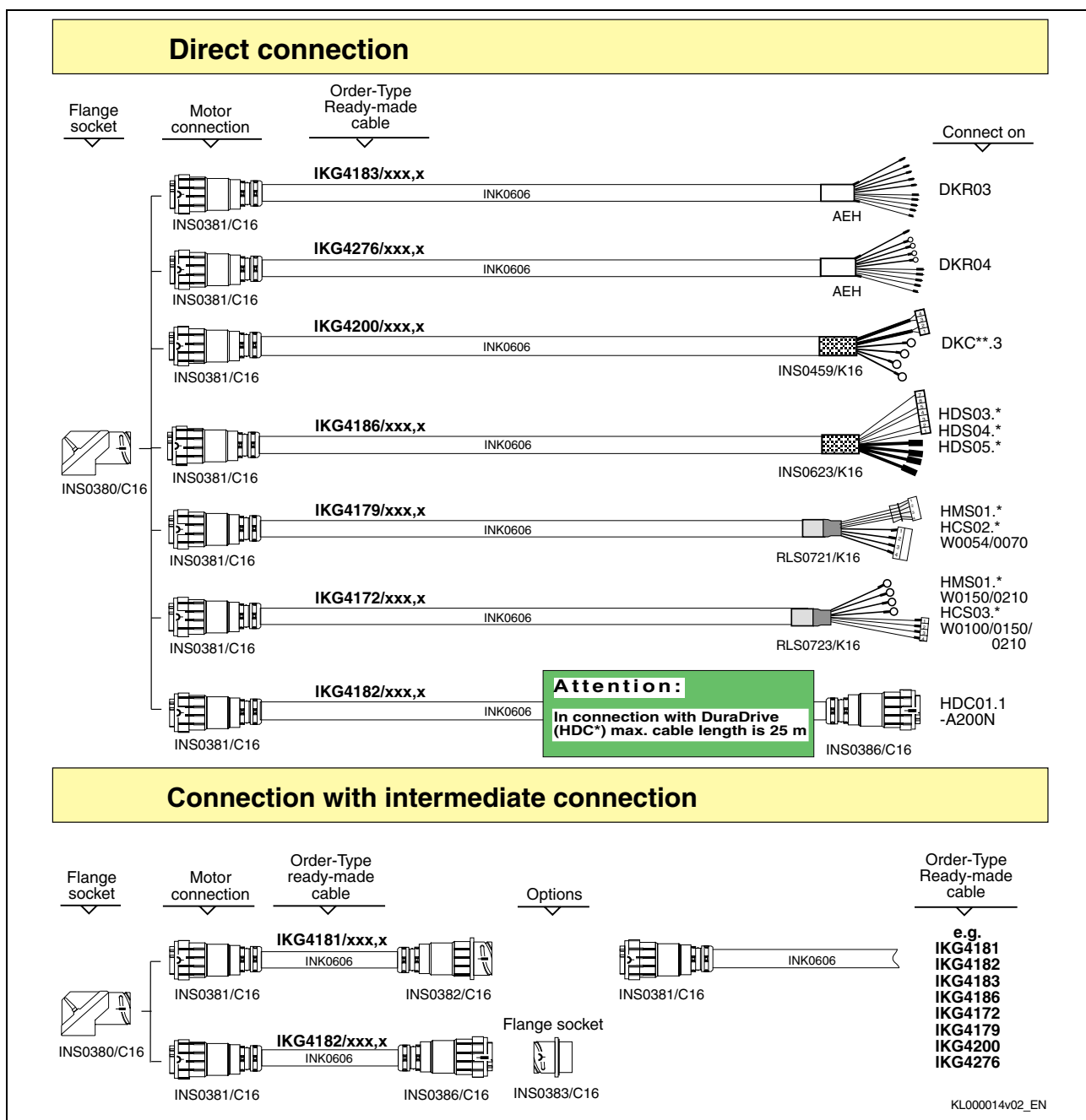
Fig. 17-11: Kabelauswahl INS0380 – 16,0mm 2
