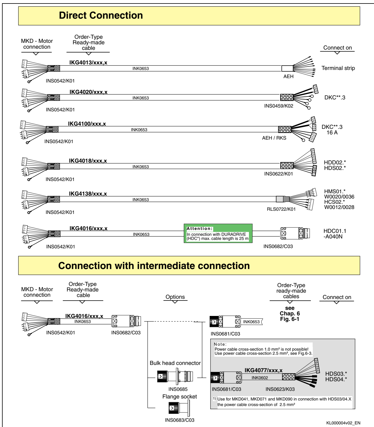
Fig. 17-3: Kabelauswahl INS0542 – 1,0mm 2
