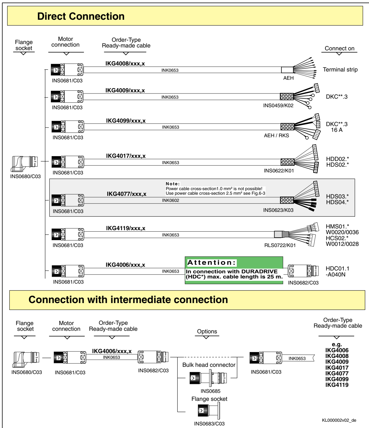
Fig. 17-2: Kabelausswahl INS0680 – 1,0mm 2
