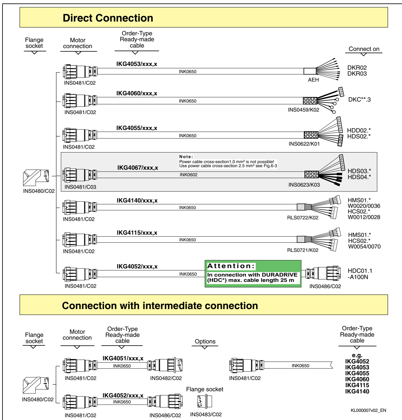
Fig. 17-4: Kabelauswahl INS0480 – 1,5mm 2
