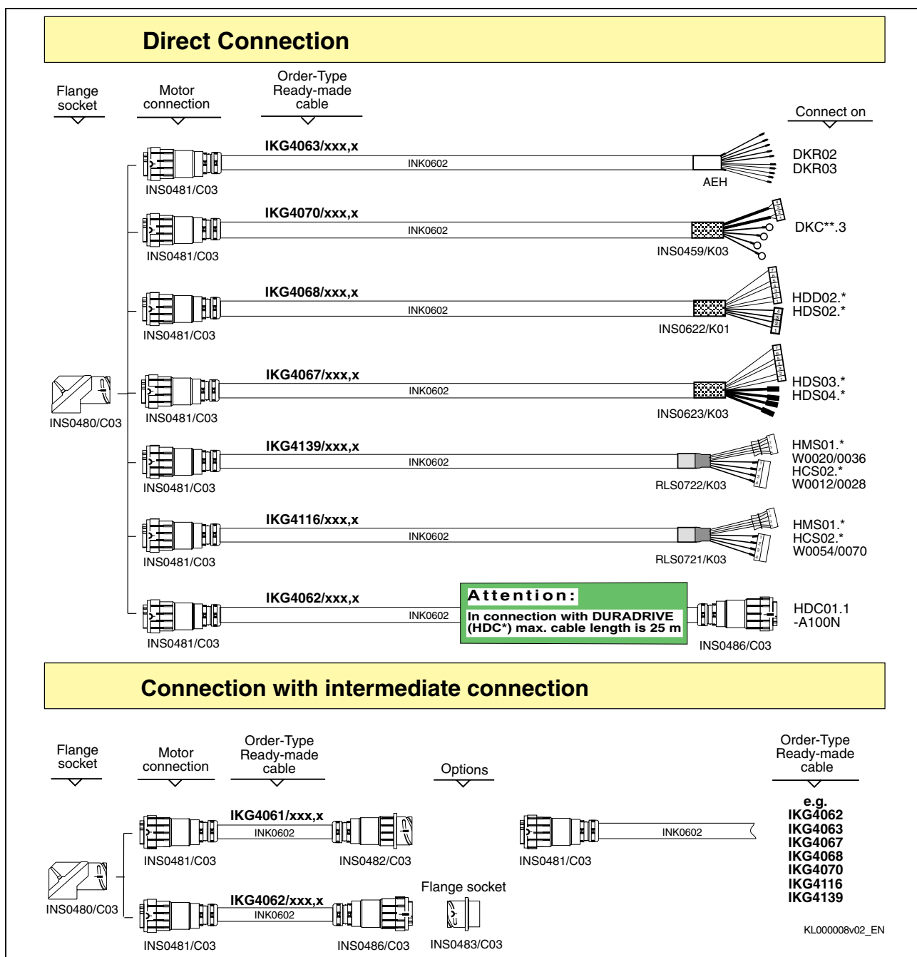
Fig. 17-5: Kabelauswahl INS0480 – 2,5mm 2
