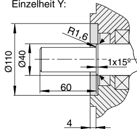
Einzelheit Y:
